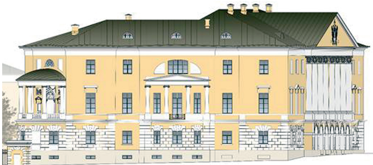
Рис. 12. Северный фасад главного дома усадьбы Мусиных-Пушкиных по Спартаковской улице в Москве. Графическая реконструкция на V строительный период (последняя треть XIX в.). Реконструкция Т.В. Иванцыка. НИИП НИУ МГСУ
