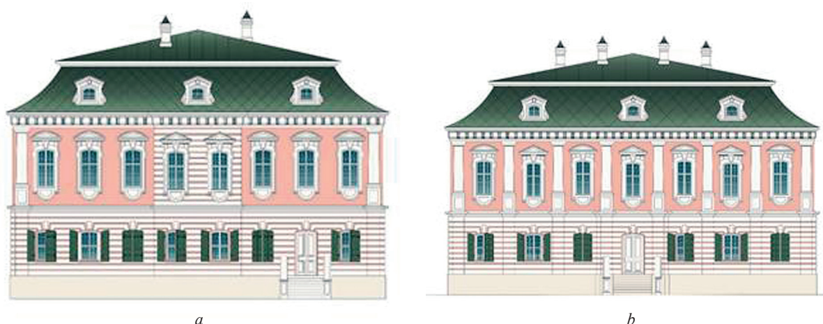
Рис. 1. Дом Д.А. Шепелева, существовавший на месте главного дома усадьбы Мусиных-Пушкиных на Спартаковской (Елоховской) улице в Москве: a — северный фасад; b — восточный фасад. Графическая реконструкция на I строительный период (середина XVIII в.). Реконструкция Т.В. Иванцыка. НИИП НИУ МГСУ
