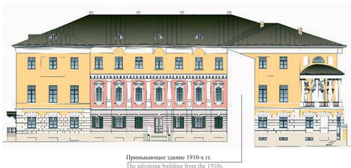
Рис. 7. Восточный фасад главного дома усадьбы Мусиных-Пушкиных по Спартаковской улице в Москве. Графическая реконструкция на V строительный период (последняя треть XIX в.) с архитектурным раскрытием I строительного периода, восточной стены дома Д.А. Шепелева (середина XVIII в.). Реконструкция Т.В. Иванцыка. НИИП НИУ МГСУ Fig. 7. The eastern facade of the main house of the Musin-Pushkin Estate in Spartakovskaya Street in Moscow. Graphical reconstruction of the 5th construction period (the last quarter of XIX c.) with architectural probe, representing 1st construction period, an eastern wall of the D.A. Shepelev's house (middle XVIII c.). Reconstruction by T.V. Ivantsyk. NIIP NRU MGSU
