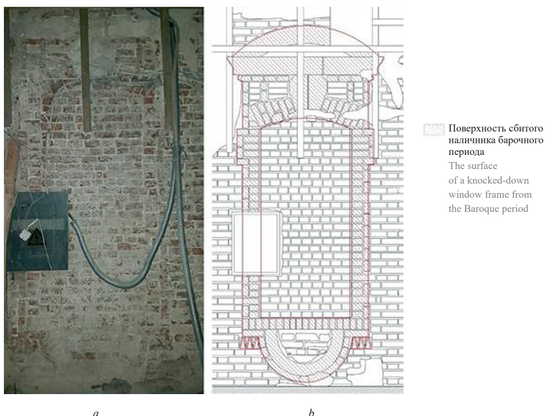
Рис. 8. Главный дом усадьбы Мусиных-Пушкиных по Спартаковской улице в Москве: a — зондаж по второму ярусу северного фасада дома Д.А. Шепелева, срубленный оконный наличник (фото 2022 г.); b — фиксация зондажа по второму ярусу северного фасада дома Д.А. Шепелева Fig. 8. The main house of the Musin-Pushkin Estate in Spartakovskaya Street in Moscow: a — probing at the 2nd tier of the northern facade of the Shepelev's house, cutted window frame (photo 2022); b — recording of the probing at the 2nd tier of the northern facade of the Shepelev's house
