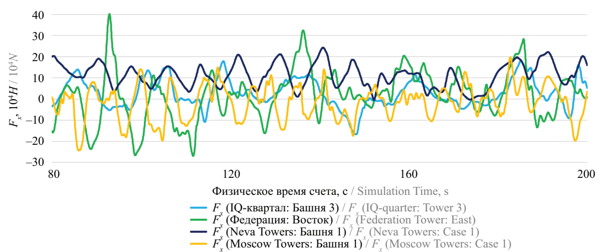
Рис. 10. Аэродинамическая сила F_x Fig. 10. Aerodynamic force F_x
