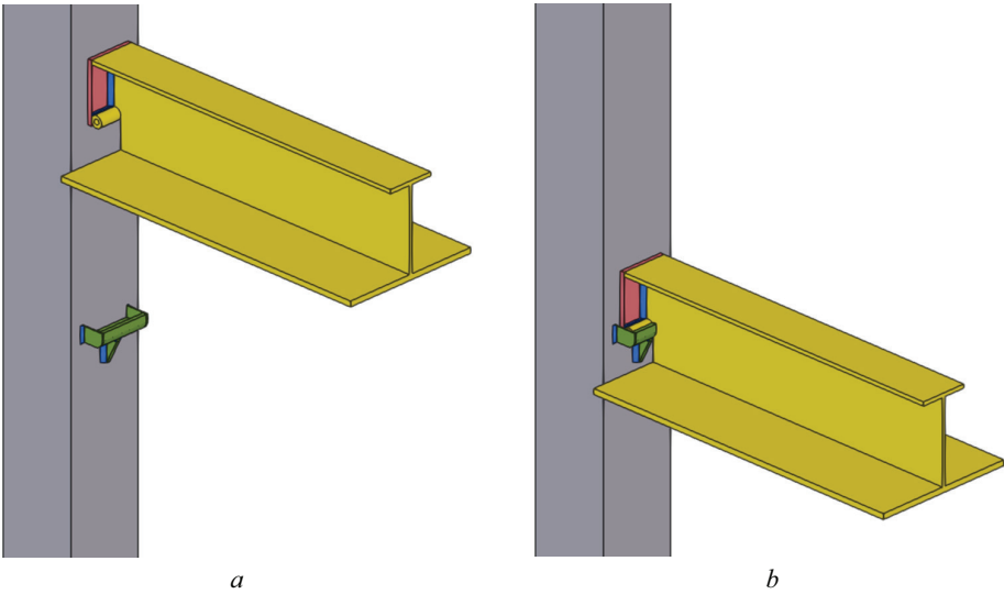
Рис. 10. Соединение стальной колонны и балки с помощью отрезка круглой трубы и гнутой пластины, формирующей «карман»: a — в разобранном виде; b — в собранном виде
