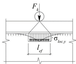
Рис. 9. Расчетная длина распределения усилия Fig. 9. Estimated length of force distribution
