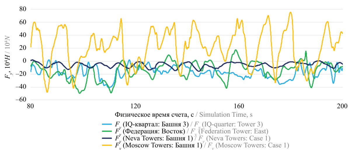
Рис. 11. Аэродинамическая сила F_y Fig. 11. Aerodynamic force F_y
