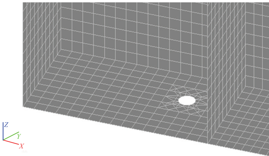
Рис. 7. Моделируемое отверстие под постоянные крепежные болты
