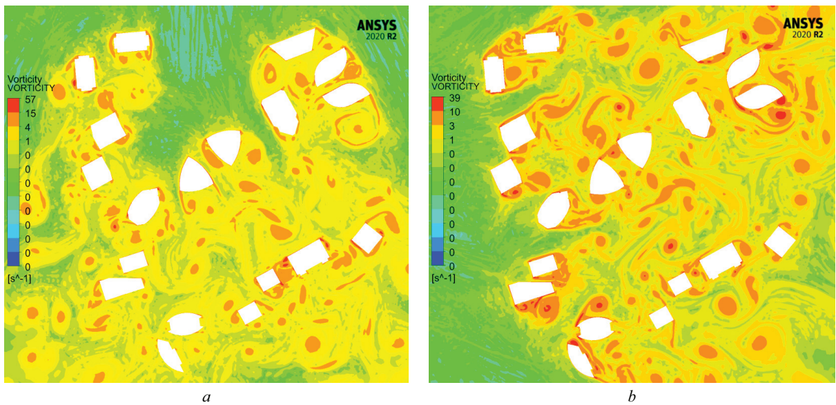
Рис. 14. Завихренности при физическом времени T = 200 с: a — северный ветер (угол атаки ветра 0^\circ ); b — западный ветер (угол атаки ветра 270^\circ ) Fig. 14. Vortices at simulation time T = 200 s: a — north wind (wind attack angle 0^\circ ); b — west wind (wind attack angle 270^\circ )
