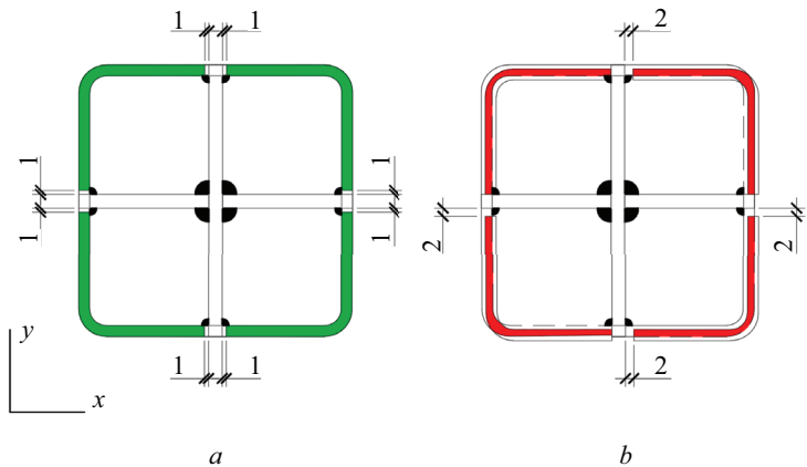
Рис. 8. Площади контакта нижней и верхней колонн: a — при идеально ровной установке; b — при перекосе Fig. 8. The contact areas of the lower and upper columns: a — in case of perfectly level installation; b — in case of misalignment
