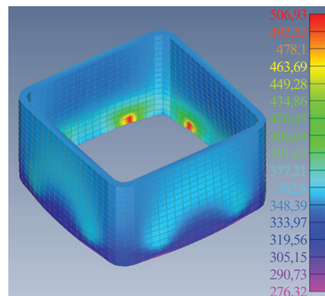
Рис. 17. Деформированный вид нижней части верхней колонны с изополями эквивалентных напряжений (1-е нагружение)
