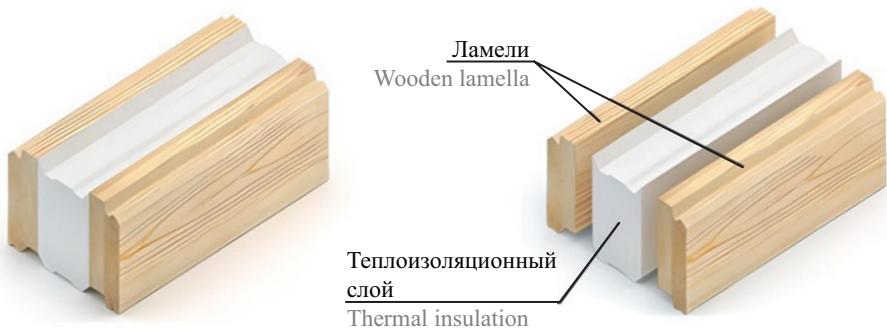
Рис. 1. Термобрус (общий вид) Fig. 1. Thermal timber (general view)
