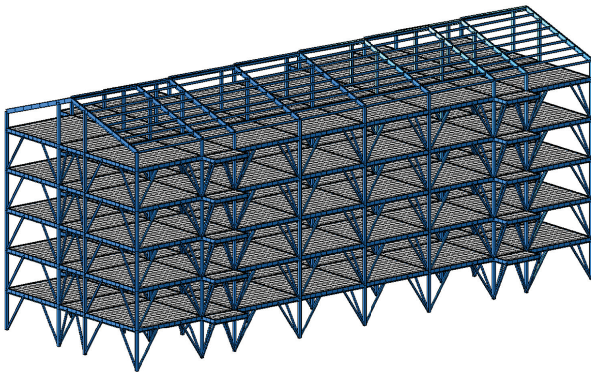
Рис. 1. Пространственная расчетная модель каркасного здания, состоящего из ячеек 6 \times 6 , 3 \times 6 и 6 \times 6 м
