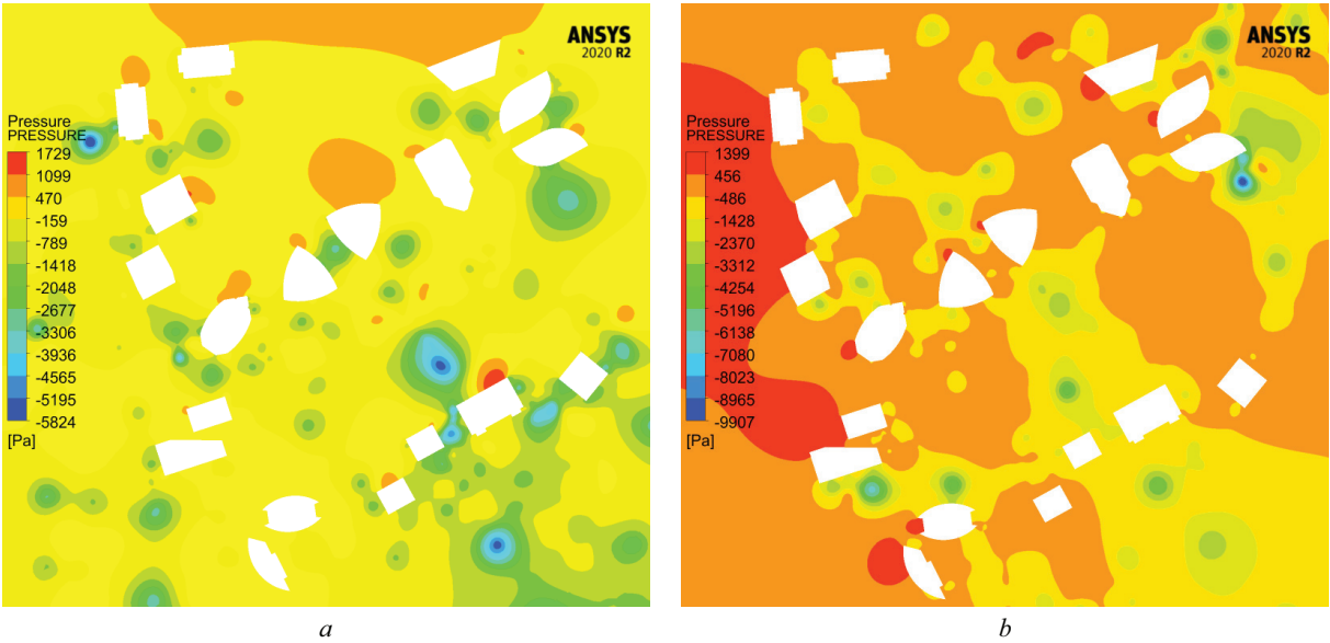
Рис. 12. Статическое давление при физическом времени T = 200 с: a — северный ветер (угол атаки ветра 0^\circ ); b — западный ветер (угол атаки ветра 270^\circ )
