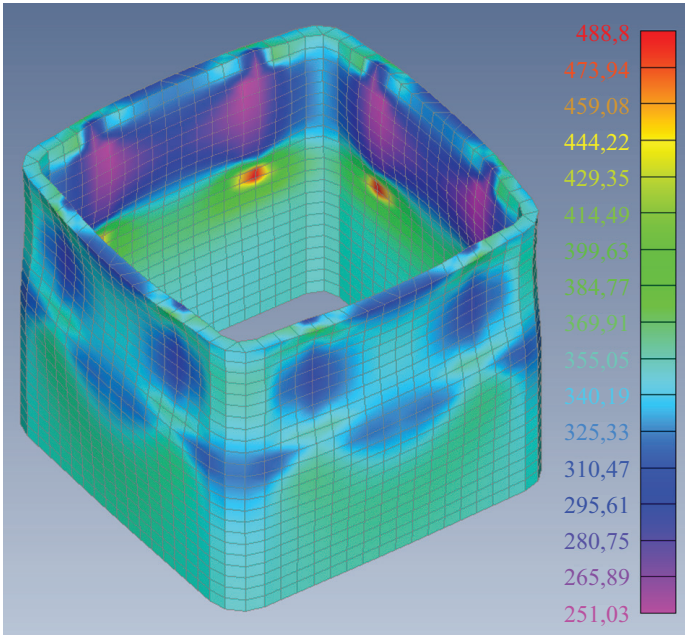
Рис. 14. Деформированный вид верхней части нижней колонны с изополями эквивалентных напряжений (1-е нагружение) Fig. 14. Deformed view of the upper part of the lower column with isofields of equivalent stresses (1st load)
