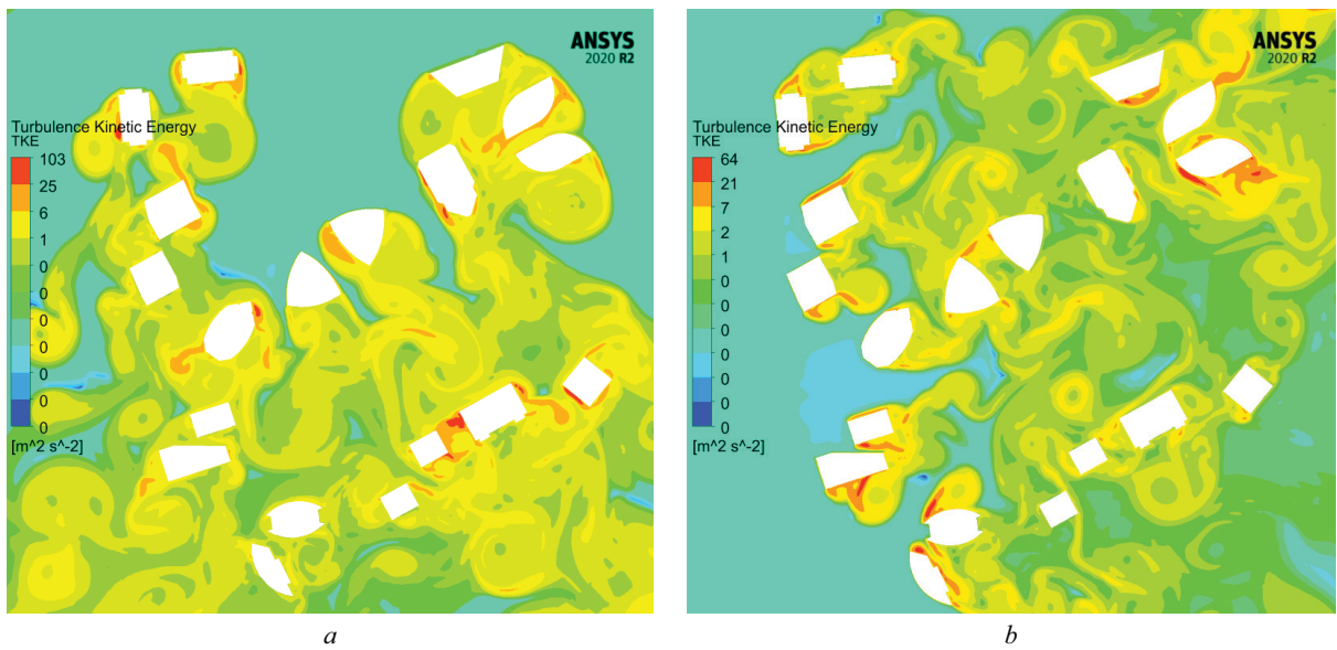
Рис. 15. Кинетическая энергия турбулентности при физическом времени T = 200 с: a — северный ветер (угол атаки ветра 0^\circ ); b — западный ветер (угол атаки ветра 270^\circ ) Fig. 15. Turbulence kinetic energy (TKE) at simulation time T = 200 s: a — north wind (wind attack angle 0^\circ ); b — west wind (wind attack angle 270^\circ )
