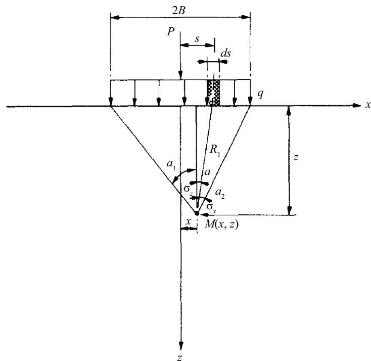
Рис. 4. Схема определения НДС с вертикальной нагрузкой, приходящей на плитный фундамент [17] Fig. 4. Scheme for determining the stress-strain state with vertical load applied to the slab foundation [17]
