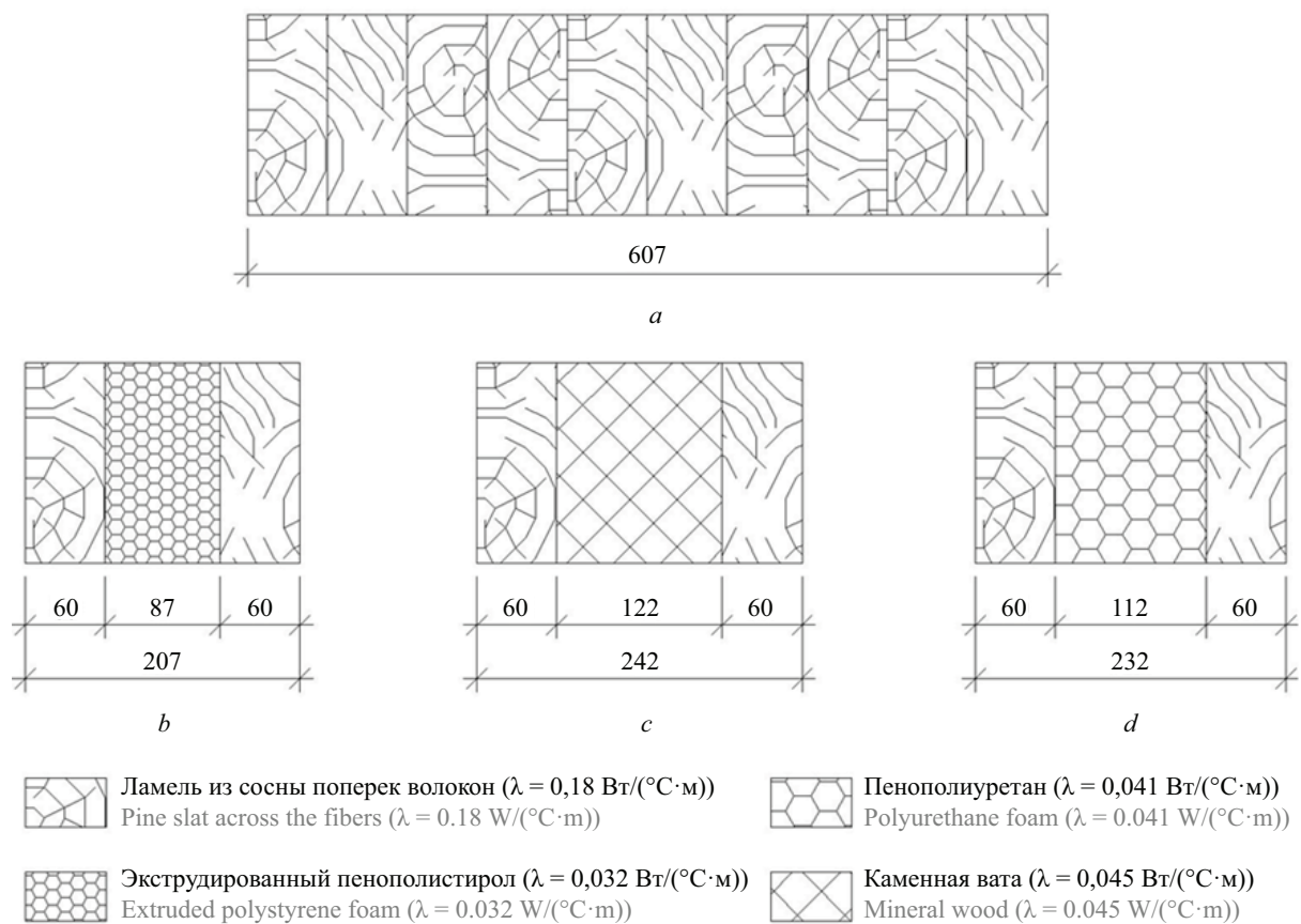
Рис. 4. Результаты теплотехнического расчета клееного бруса (a) и термобруса с разными теплоизоляционными материалами: b — экструдированный пенополистирол; c — каменная вата; d — пенополиуретан Fig. 4. The results of thermal calculation of the glued timber (a) and the thermal timber made with different heat-insulating materials: b — extruded polystyrene foam; c — mineral wool; d — polyurethane foam
