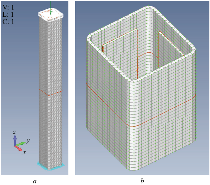
Рис. 11. Конечно-элементная модель узла стыка колонн с использованием пластин: a — общий вид; b — узел стыка крупным планом
