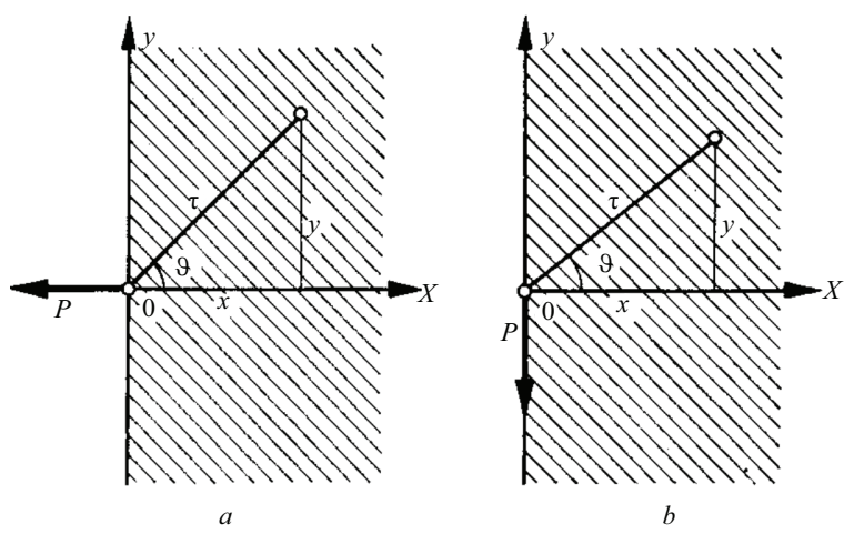
Рис. 2. Схема определения НДС при сосредоточенной нагрузке P на границе полупространства, действующей перпендикулярно (а) и параллельно (б) ограниченному краю полупространства [15]
