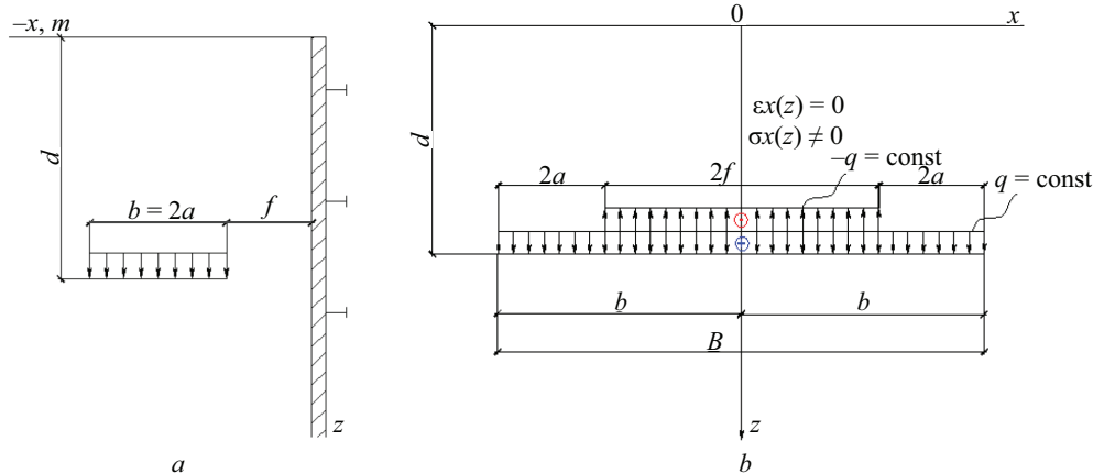
Рис. 6. Итоговый вид нагрузки на глубине для определения НДС основания (а); схема определения нагрузки для расчета НДС (b) [19]
