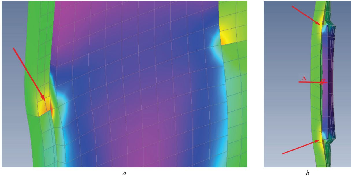
Рис. 16. Увеличенный вид контакта пластины и стенки трубы (а) и вид сверху (b) для 1-го нагружения
