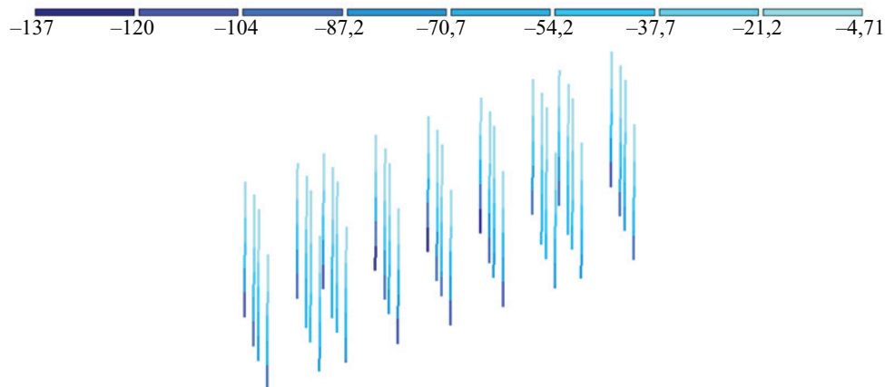
Рис. 4. Мозаика продольных сил N , т, в колоннах
