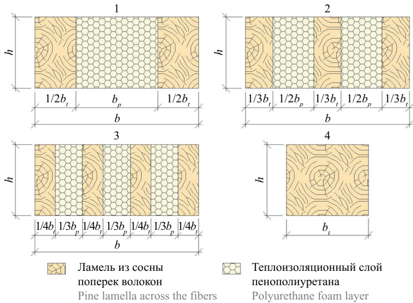
Рис. 3. Поперечное сечение лабораторных образцов для проведения испытаний
