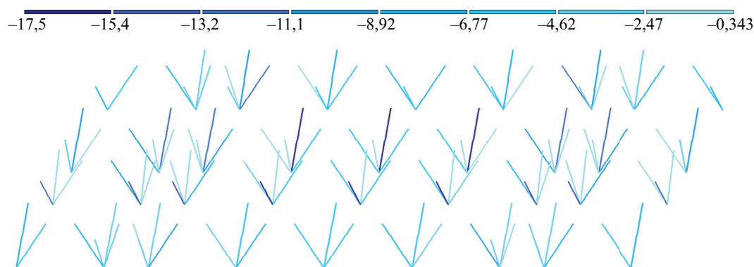
Рис. 5. Мозаика продольных сил N , t , в подкосах первого этажа
