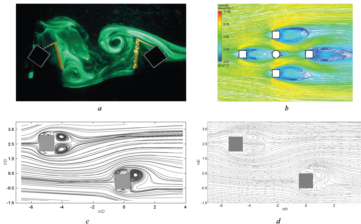
Рис. 1. Визуализация влияния периодических вихревых структур на здание, расположенное в аэродинамическом следе (a) [2]; линии тока при угле атаки ветра 0° (b) [3]; усредненные по времени линии тока на средней высоте: результат LES-моделирования (c) и результат эксперимента в аэродинамической трубе (d) [4]
