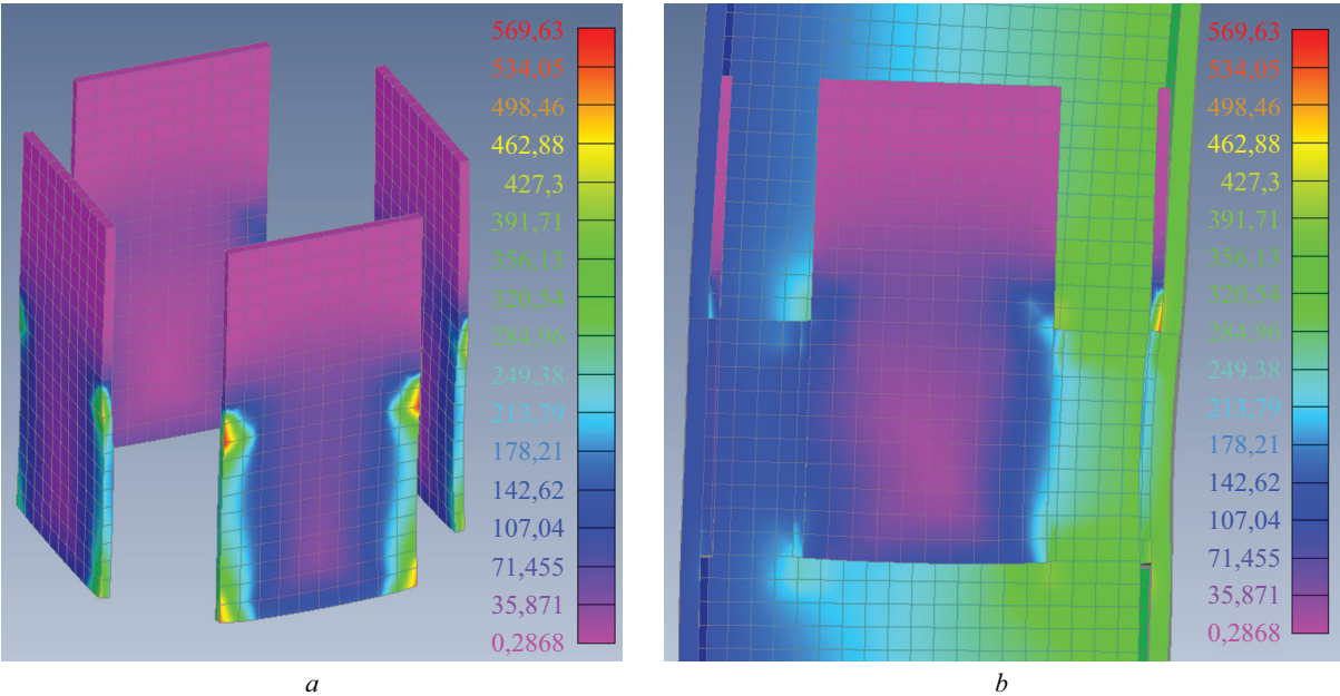
Рис. 20. Деформированный вид пластин с изополями эквивалентных напряжений (а) и разрез по узлу (b) для 2-го нагружения
