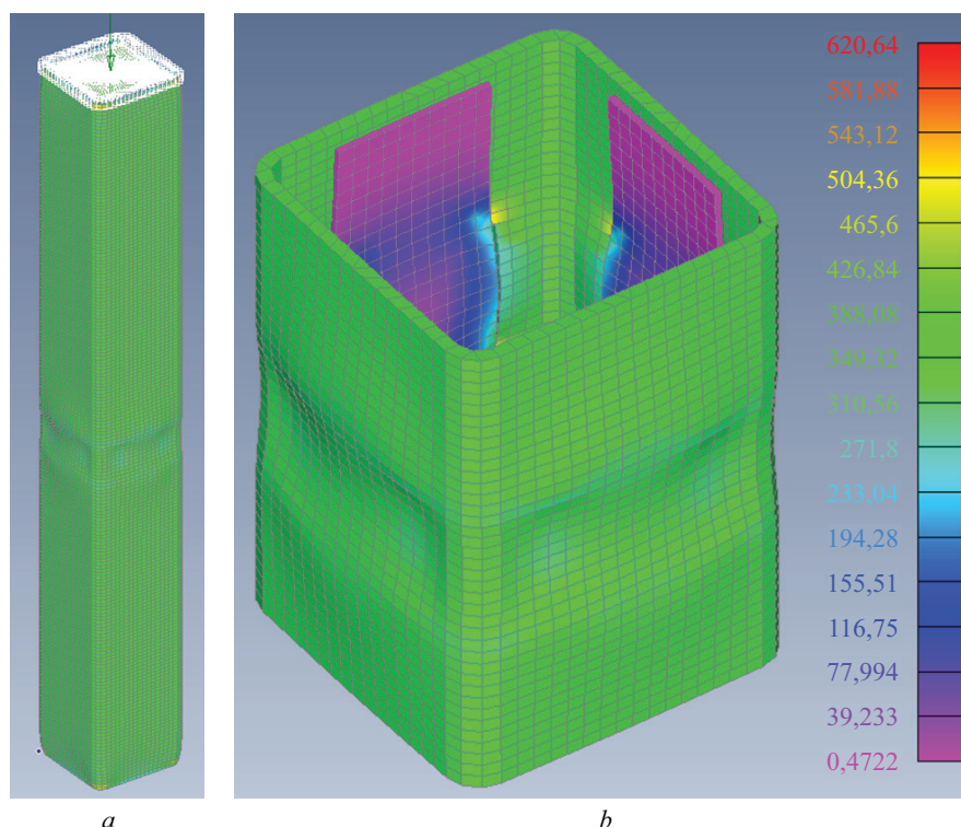
Рис. 12. Деформированный вид модели с изополями эквивалентных напряжений (1-е нагружение): a — общий вид; b — узел стыка крупным планом
