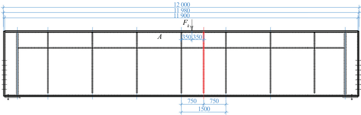
Рис. 11. Схема балки с установкой дополнительных ребер жесткости
