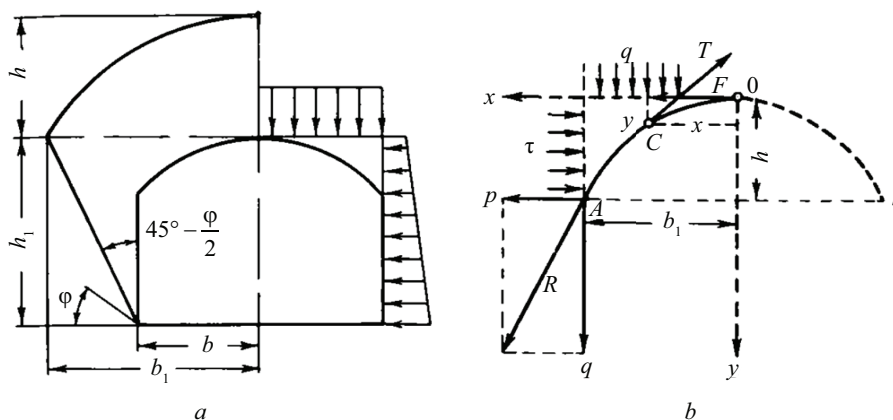
Рис. 1. Схема давления породы по М.М. Протодяконову [3]
