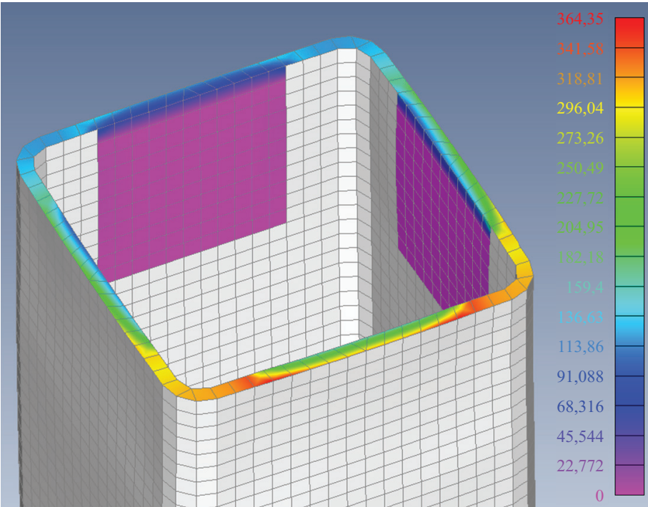
Рис. 21. Изополе нормальных контактных напряжений на торце трубы (2-е нагружение)
