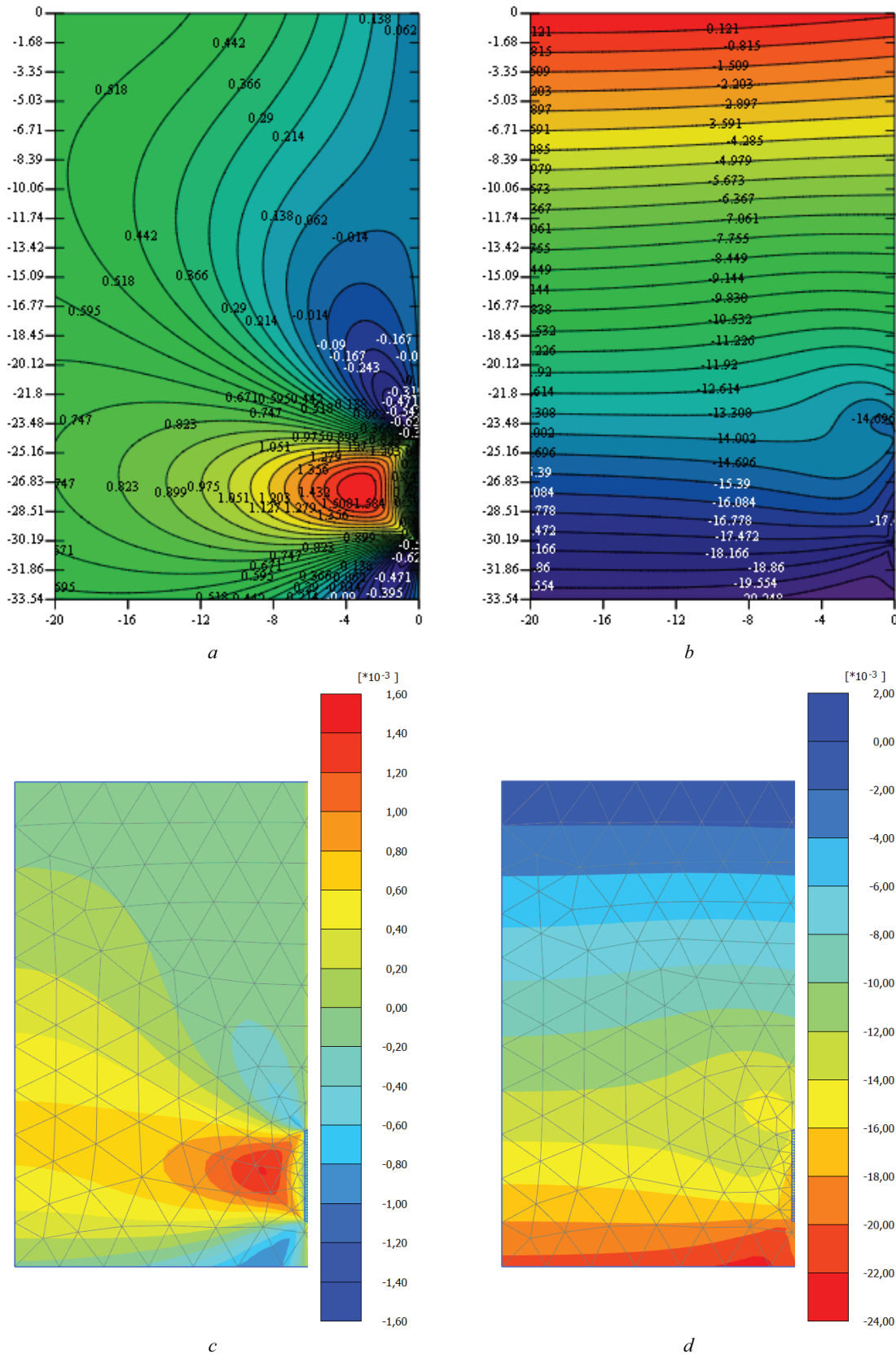
Рис. 10. Изополя вертикальных деформаций \epsilon_z при приложении давления пригруза к массиву: деформации без учета веса грунта, полученные в MathCad (a); деформации с учетом веса грунта, полученные в MathCad (b); деформации без учета веса грунта, полученные в Plaxis 2D (c); деформации с учетом веса грунта, полученные в Plaxis 2D (d)
