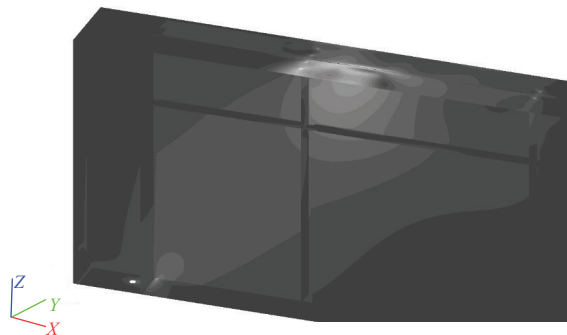
Рис. 13. Иллюстрация изополей напряжений в элементах ПБ при промежуточном положении нагрузки в отсеке с эксцентриситетом e = 25 мм (промежуточное положение крановой нагрузки в пролете балки)
