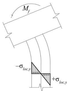
Рис. 8. Схема распределения нормальных напряжений при кручении пояса балки Fig. 8. The scheme of distribution of normal stresses during torsion of the beam belt
