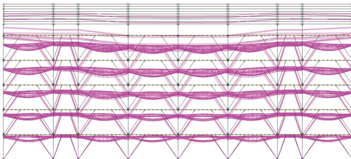
Рис. 2. Деформированный вид расчетной схемы здания
