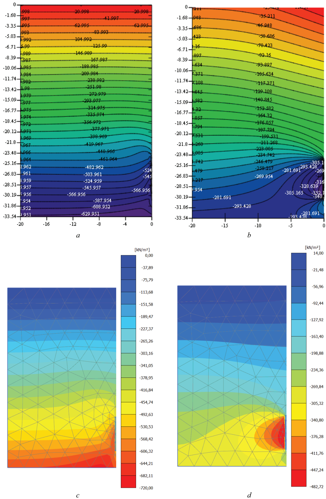
Рис. 9. Изополя напряжений при приложении давления пригруза к грунтовому массиву с учетом напряжений от собственного веса грунта \gamma_h : вертикальные напряжения P_z , полученные в MathCad (a); горизонтальные напряжения P_x , полученные в MathCad (b); вертикальные напряжения P_z , полученные в Plaxis 2D (c); горизонтальные напряжения P_x , полученные в Plaxis 2D (d)
