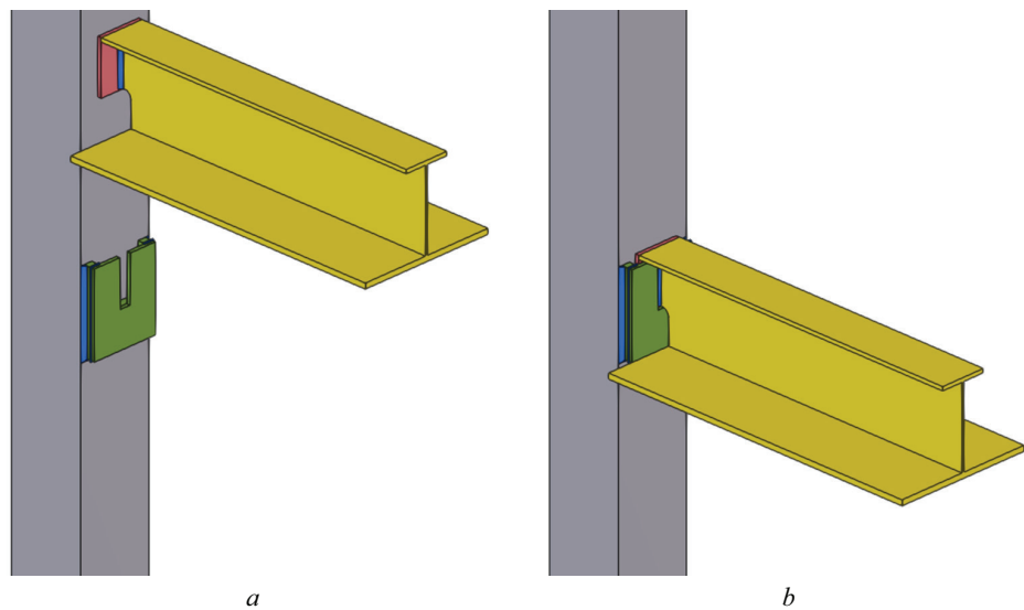
Рис. 9. Соединение стальной колонны и балки по системе «ласточкин хвост»: a — в разобранном виде; b — в собранном виде
