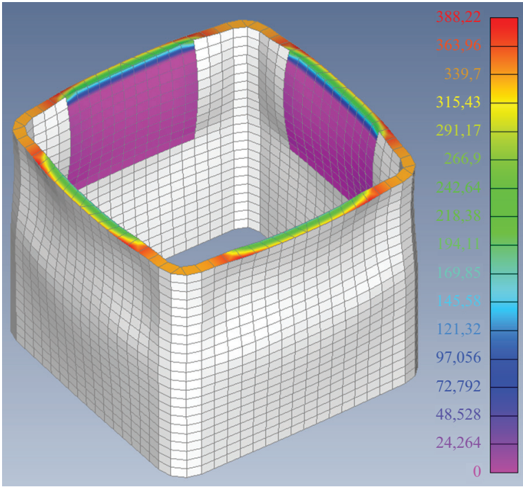
Рис. 18. Изополе нормальных контактных напряжений на торце трубы (1-е нагружение) Fig. 18. Isofield of normal contact stresses at the end of the pipe (1st load)
