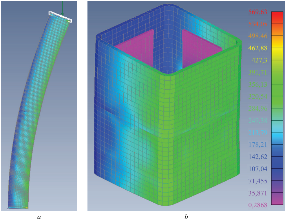
Рис. 19. Деформированный вид модели с изополями эквивалентных напряжений (2-е нагружение): a — общий вид; b — узел стыка крупным планом Fig. 19. Deformed view of the model with isofields of equivalent stresses (2nd load): a — general view; b — close-up of the junction
