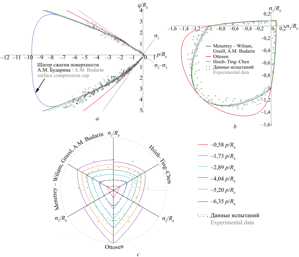
Рис. 15. Сравнение поверхностей четвертой группы с результатами опытов: меридиональное сечение (а); сечение \sigma_1-\sigma_3 (b); девиаторные сечения (с) Fig. 15. Comparison of the surfaces of the fourth group with the results of experiments: meridional section (a); section \sigma_1-\sigma_3 (b); deviatoric section (c)
