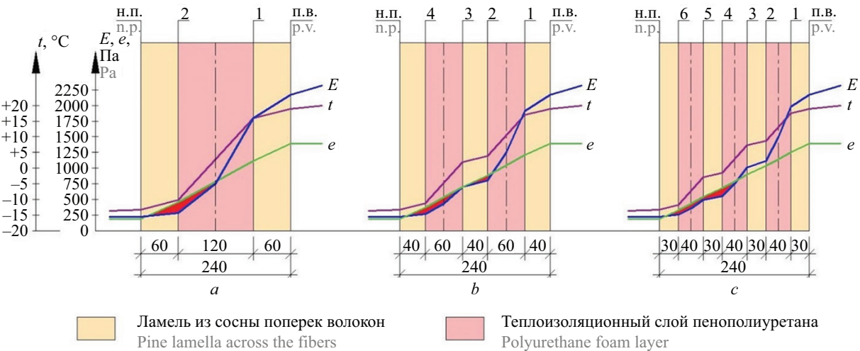
Рис. 5. Графики распределения температуры t и парциального давления водяного пара E и e по толще термобруса с разными вариантами чередования слоев
