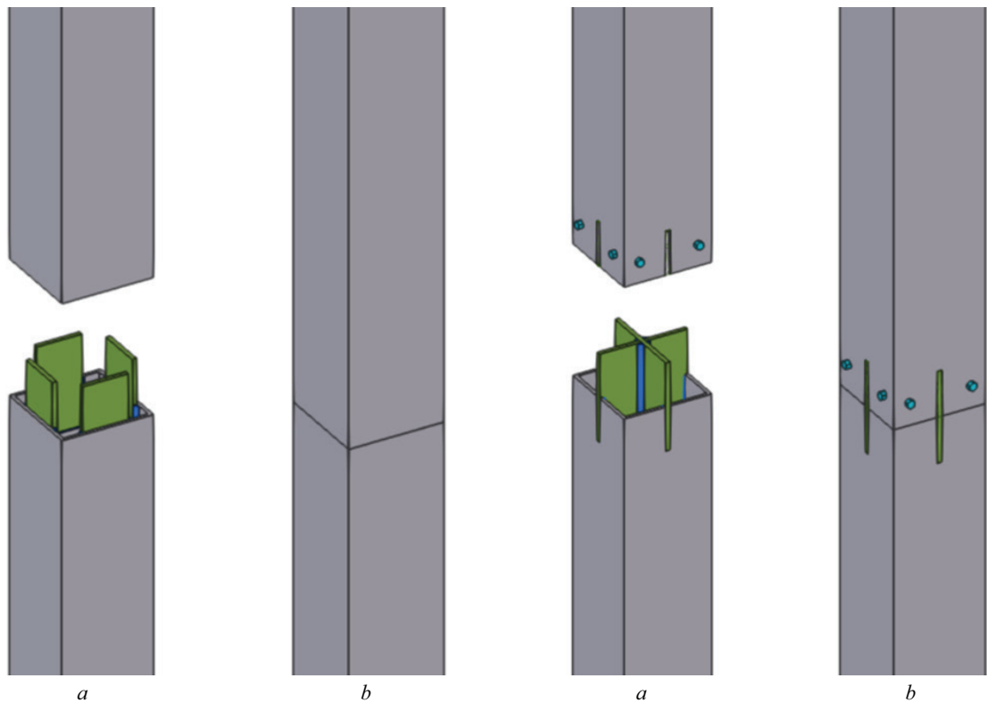
Рис. 7. Контактный стык колонн сечением из квадратных труб с направляющей сварной крестовиной: a — в разобранном виде; b — в собранном виде
