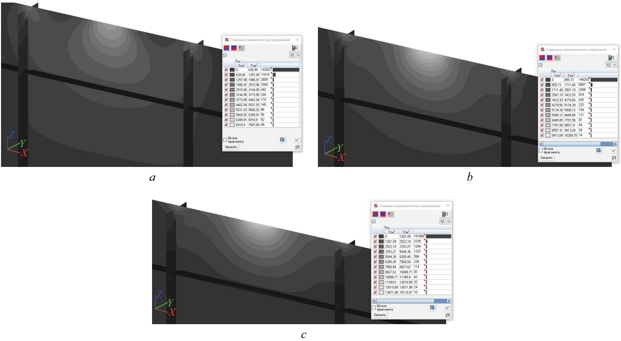
Рис. 16. Нагрузка в середине отсека с эксцентриситетом: а — e = 0 мм; б — e = 25 мм; с — e = 50 мм (в середине пролета балки) Fig. 16. Load in the middle of the compartment with eccentricity of: а — e = 0 mm; б — e = 25 mm; с — e = 50 mm (in the middle of the beam span)
