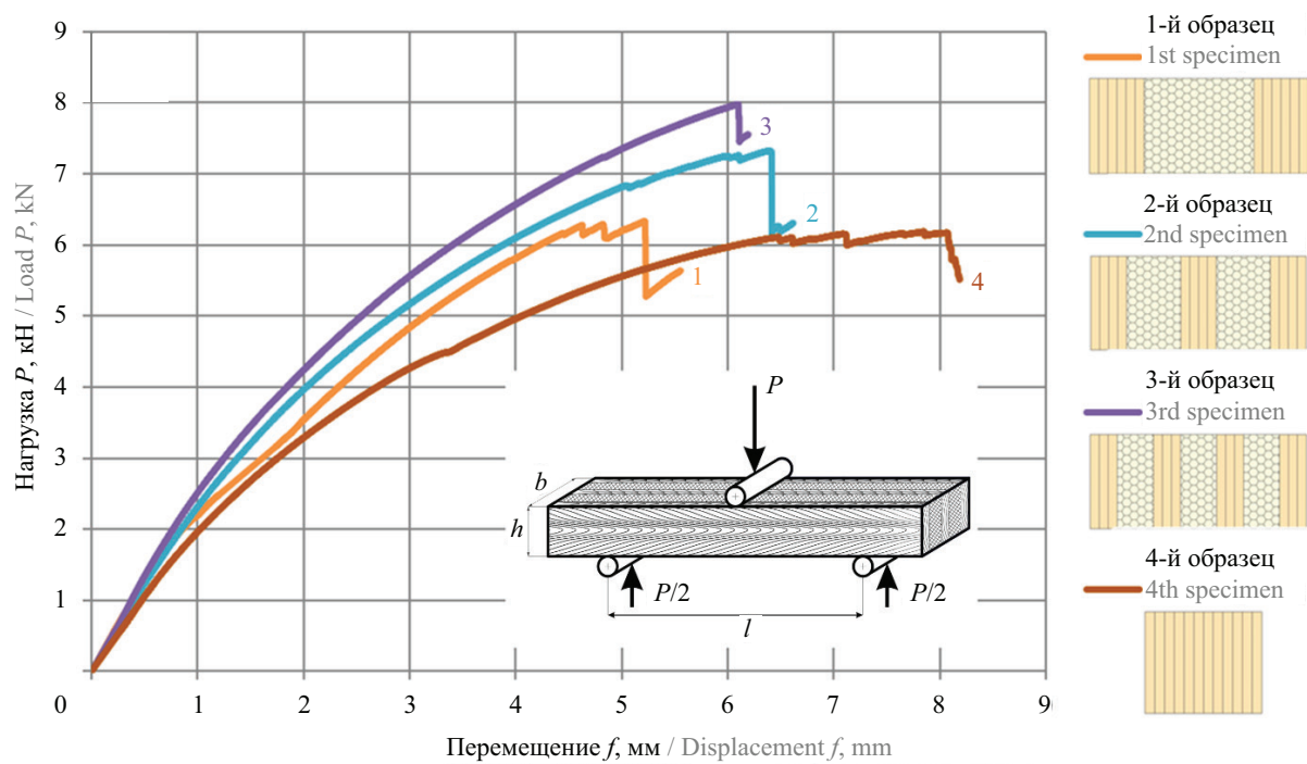
Рис. 6. Результаты эксперимента и схема проведения испытаний на поперечный изгиб Fig. 6. Experimental results and scheme of cross-bending tests
