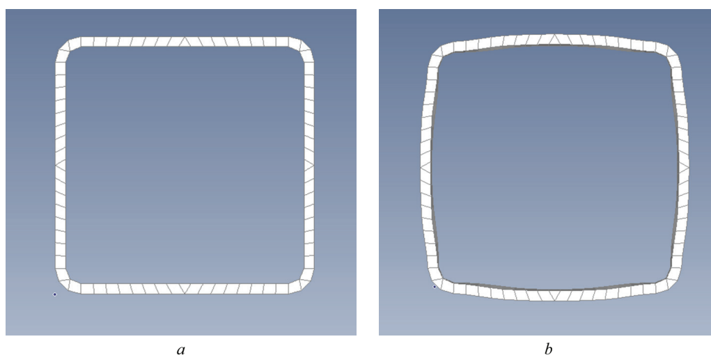
Рис. 13. Форма колонны: a — до деформации; b — после деформации (1-е нагружение)
