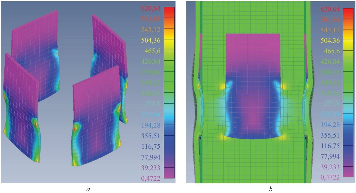
Рис. 15. Деформированный вид пластин с изополями эквивалентных напряжений (а) и разрез по узлу (b) для 1-го нагружения Fig. 15. Deformed appearance of plates with isofields of equivalent stresses (a) and a section along the joint (b) for 1st load
