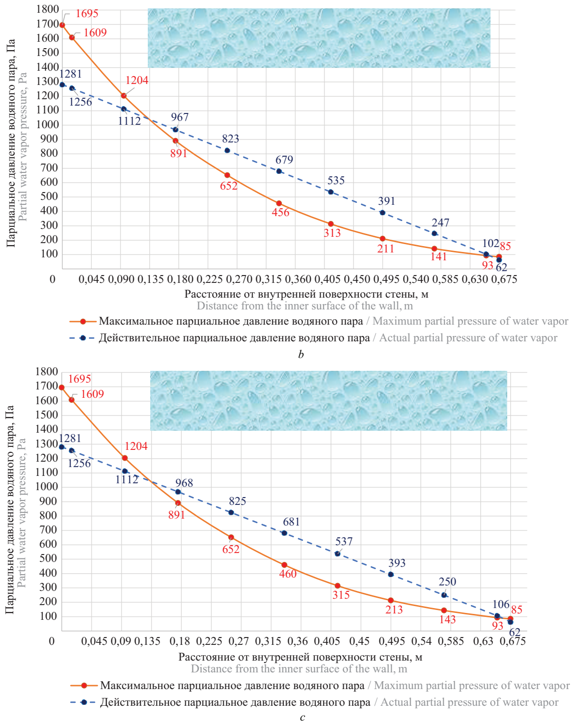
Рис. 4. Распределение парциальных давлений водяного пара по толщине стеновой конструкции с наружным штукатурным покрытием из известково-песчаного раствора (а); сложного раствора (б); цементно-песчаного раствора (с) для условий наиболее холодной пятидневки
