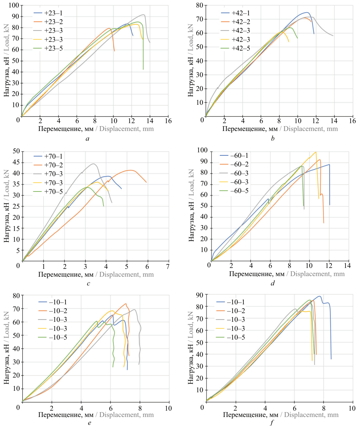
Рис. 4. Диаграммы «нагрузка – перемещение» при температуре: +23 °C (a); +42 °C (b); +70 °C (c); –60 °C (d); –10 °C (7 сут) (e); –10 °C (10 сут) (f)
