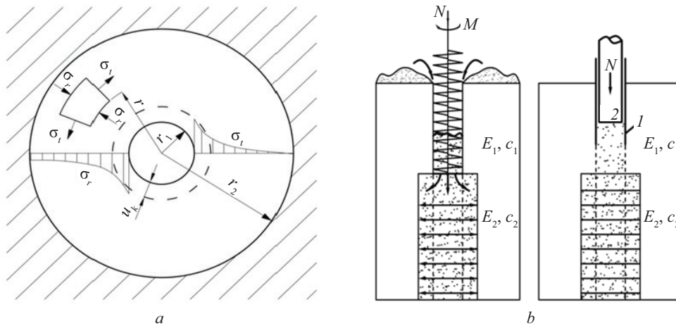
Рис. 3. Расчетная схема расширения диаметра лидирующей скважины (а) и технологии ее расширения (b) [15]: \sigma_r — радиальные напряжения; \sigma_t — тангенциальные напряжения; u_k — перемещение стенки скважины в радиальном направлении; E_1 — модуль деформации окружающего грунта; E_2 — модуль деформации колонны; C_1 — сцепление грунта; C_2 — сцепление щебня; N — ось продольных усилий; M — момент вращения рабочего органа
