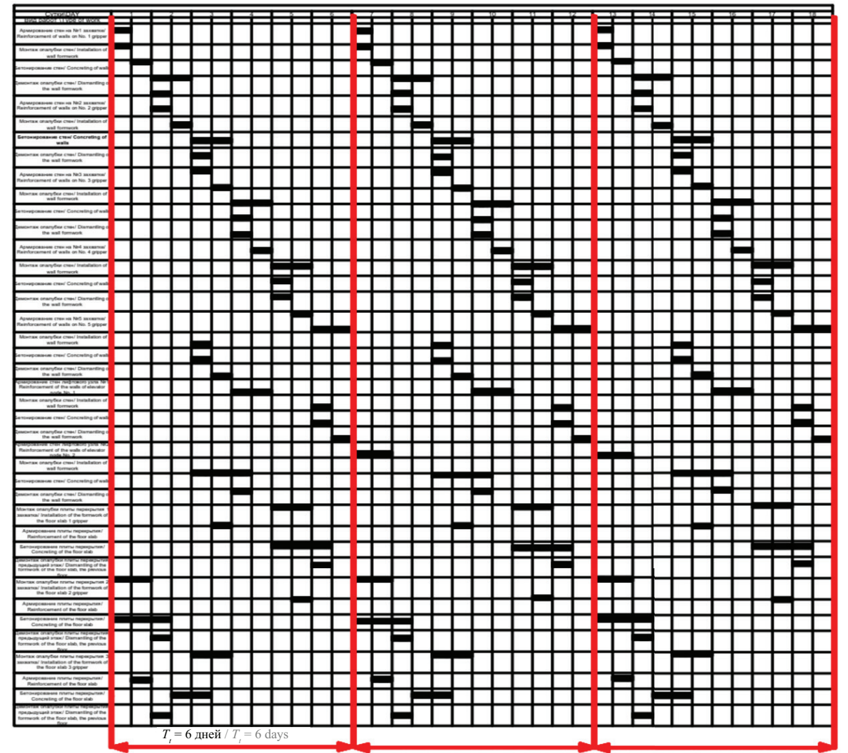
Рис. 6. Целевой график с темпом 6 дней на этаж
